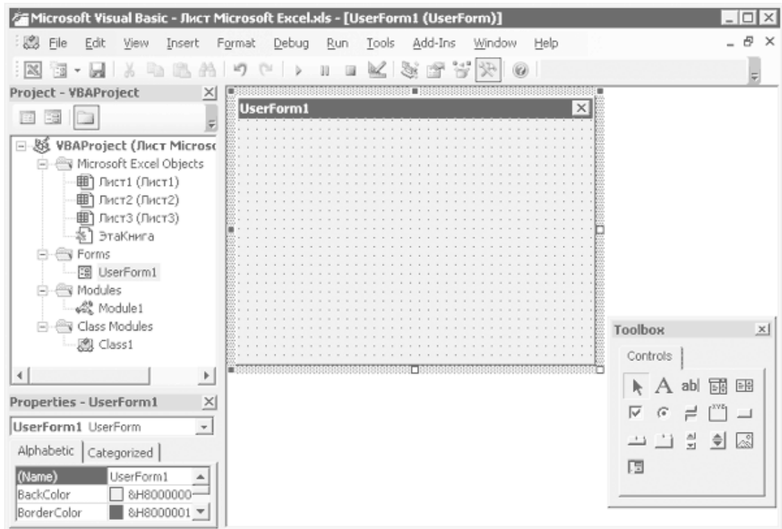
Рис. 1.2. Редактирование формы
