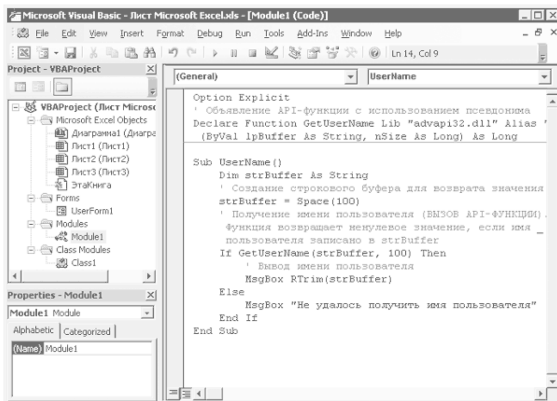
Рис. 1.1. Проект VBA
